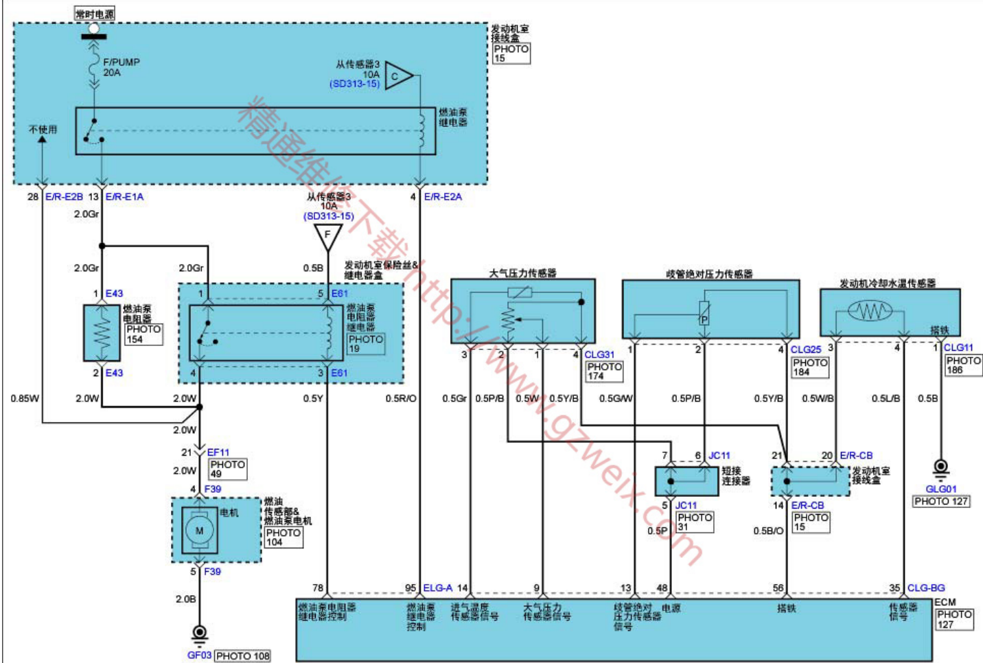
MFI 控制系统(G6DJ : LAMBDA 3.8L GDI) (5)
